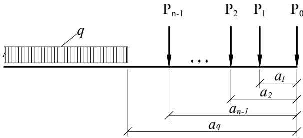
Рис. 1. Схема подвижного состава, заданная сосредоточенными силами P_0, P_1, \dots, P_{n-1} и равномерно распределенной нагрузкой интенсивности q
