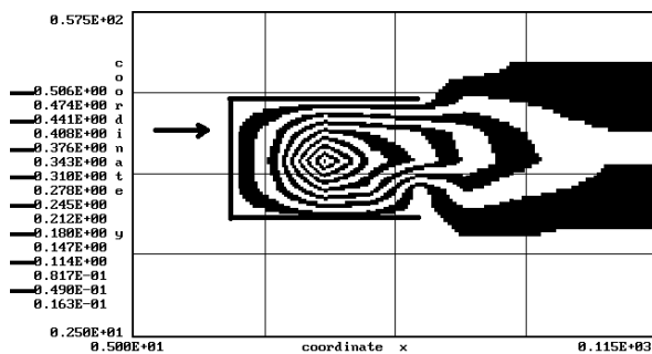
Рис. 7. Зона загрязнения атмосферы для момента времени t = 30 с (сечение z = 2,5 м)
