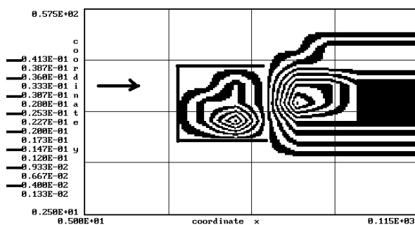
Рис. 8. Зона загрязнения атмосферы для момента времени t = 30 с (сечение z = 7,5 м)
