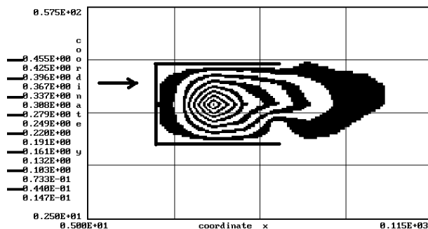
Рис. 6. Зона загрязнения атмосферы для момента времени t = 12 с (сечение z = 2,5 м)
