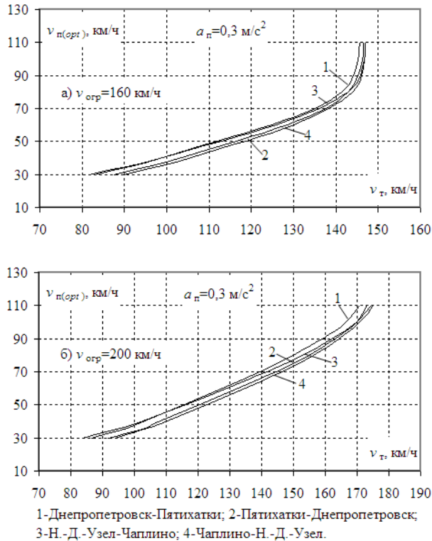
Рис. 1. Зависимость оптимальной пусковой скорости от технической для электровоза постоянного тока
