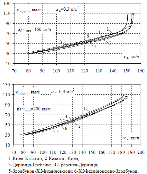
Рис. 2. Зависимость оптимальной пусковой скорости от технической для электровоза переменного тока
