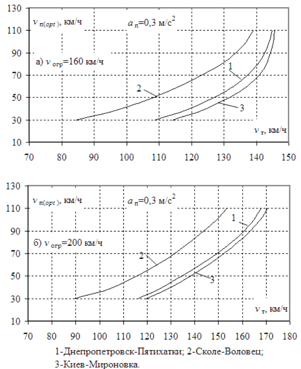
Рис. 3. Зависимость оптимальной пусковой скорости от технической для электровоза с АТП
