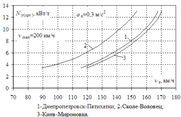
Рис. 4 – Зависимость оптимальной удельной мощности электровоза от технической скорости для электровоза с АТП
