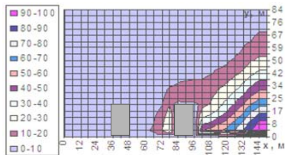
Рис. 8. Зона замітнення атмосферного воздуха для t=40 с, C_{\max}=0,061 г/м 3
