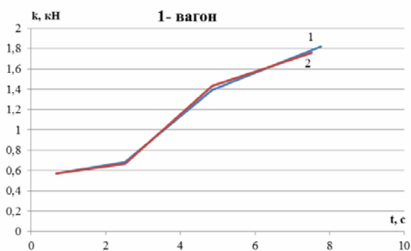
Рис. 7. Діаграма наповнення тормозного циліндра в 1-ом вагоні грузового поїзда, що складається з 60 вагонів при екстремному торможенні
