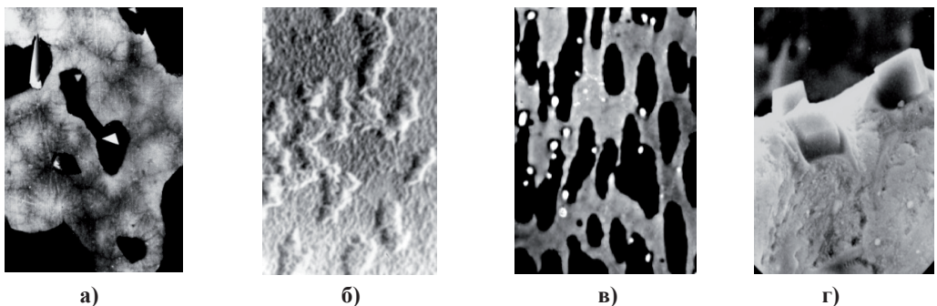
Рис. 5. Расслоение в цементите, легированном вольфрамом (а), хромом (б) и выделение карбидов WC в цементите, легированном ванадием (в, г):
