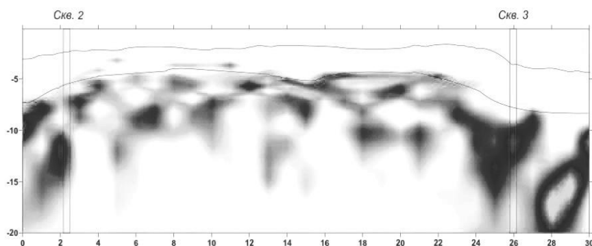
Рис. 1. Схема распределения значений напряженности поля ЕИЭМПЗ на участке исследований по глубине, м.
