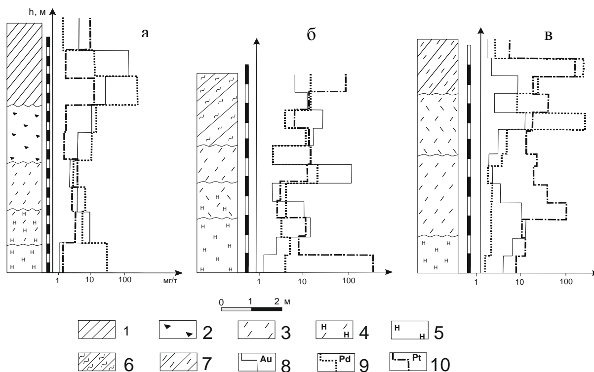
Рис. 1. Распределение благородных металлов в вертикальном разрезе нонтронитовых кор выветривания на Восточно-Липовеньковском, Западно-Липовеньковском и Капитановском месторождениях.
