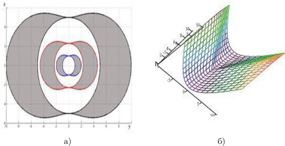
Рис. 4: Функції розподілу темної матерії: а) кількість темної матерії (сіра заливка) як функція радіусів \{r_1 = 1; r_2 = 2, 3; r_3 = 5\} та кутів 0 \leq \theta \leq 2\pi , б) ізолінії (осесиметричні ізоповерхні) розподілу темної матерії
