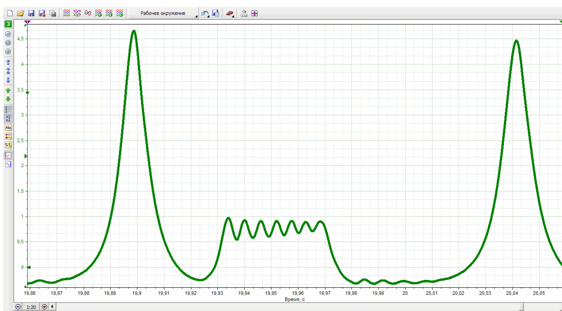
Рис.4. Осциллограмма давления в цилиндре двигателя с внутренним разрушением катализатора либо глушителя
