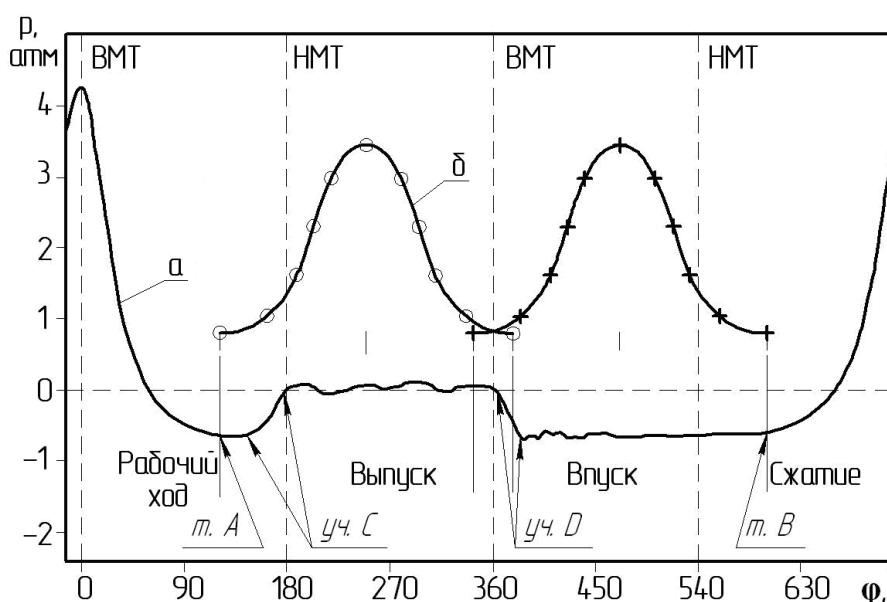
Рис. 1. Осциллограмма давления в цилиндре (норма): кривая а - осциллограмма давления; кривая б - процесс открытия и закрытия клапанов
