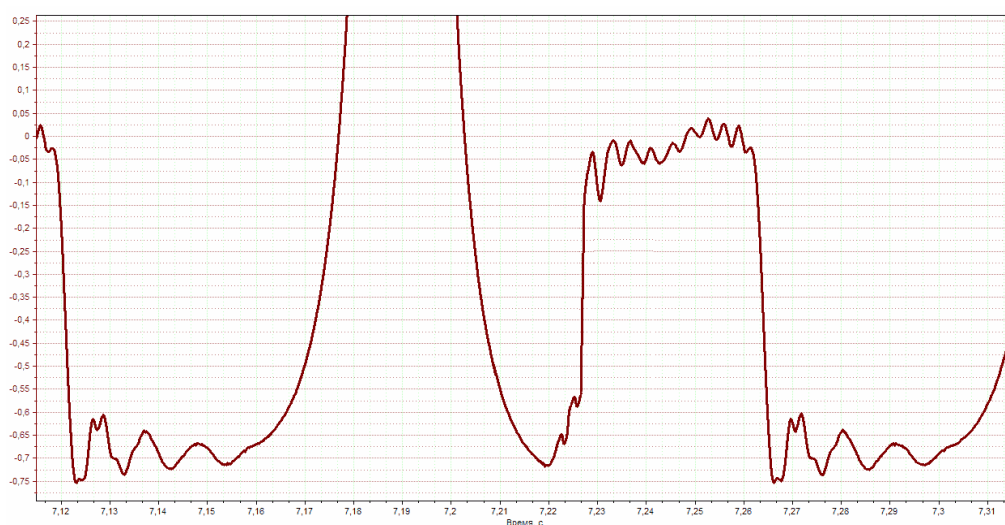
Рис. 3. Осциллограмма давления в цилиндре двигателя с изношенной клапанной втулкой
