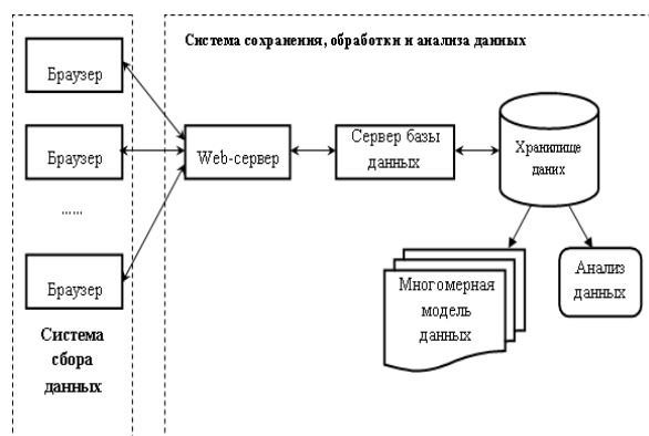
Рис. 1. Общая схема системы СУБД
