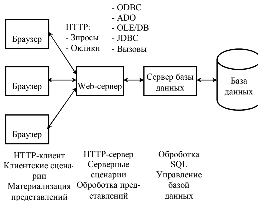
Рис. 2. Функции уровней (стандарты и интерфейсы)
