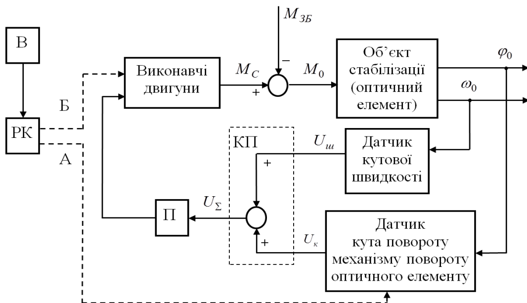
Рис. 1. Функціональна схема стабілізатора освітлення
