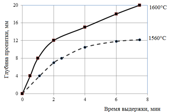
Рис. 2. Влияние температуры заливаемого металла и времени выдержки расплава на глубину пропитки
