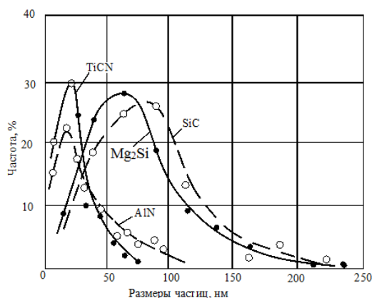
Рис. 1. Гистограмма распределения наночастиц Ti(CN), AlN, SiC, Mg 2 Si
