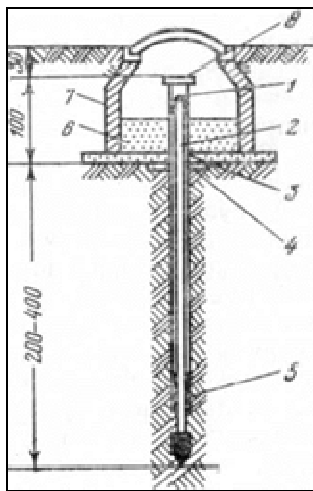
Рис. 3. Будова трубчатого ґрунтового репера: 1 – реперна головка діаметром 2–4 см; 2 – реперна труба діаметром 7–8 см; 3 – захисна труба діаметром 12–15 см; 4 – хомут для утримання захисної труби; 5 – ґрунт; 6 – шлак; 7 – цегляний або бетонний (збірний) колодязь; 8 – кришка
