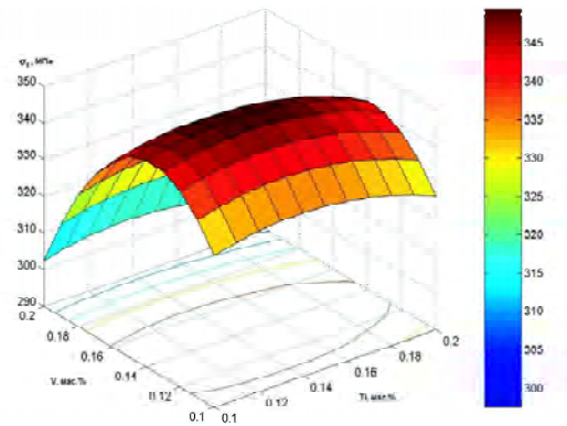
Рис. 2. Оптимизация химического состава стали по пределу текучести ( \sigma_T )
