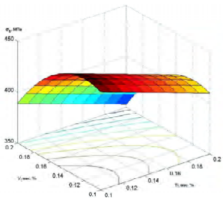
Рис. 1. Оптимизация химического состава стали по пределу прочности ( \sigma_B )
