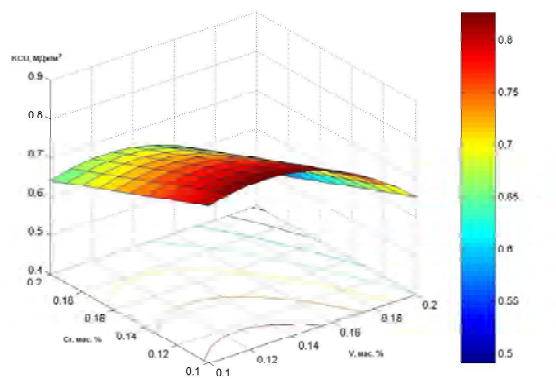
Рис. 3. Оптимизация химического состава стали по ударной вязкости
