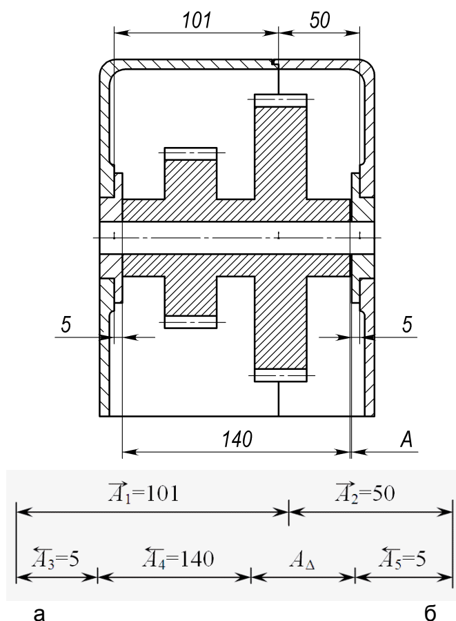
Рис. 2. Размерная цепь
