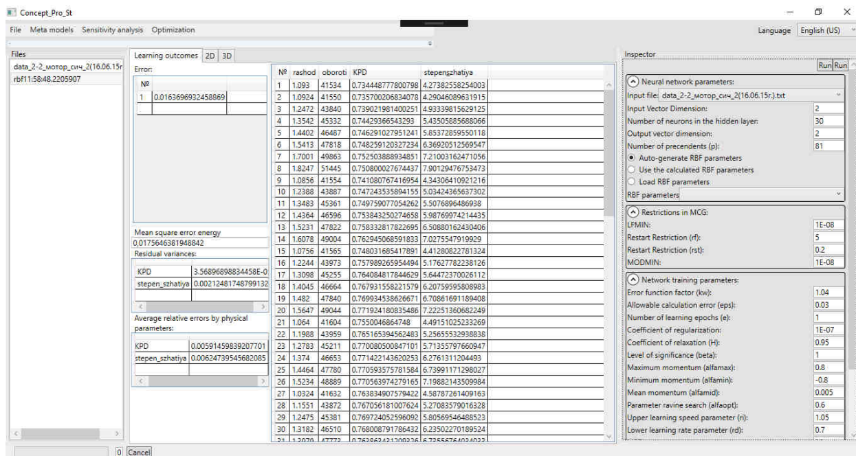
Рис. 3. Результаты робастной аппроксимации напорных характеристик многоступенчатого осевого компрессора (МОК) с помощью радиально-базисной сети
