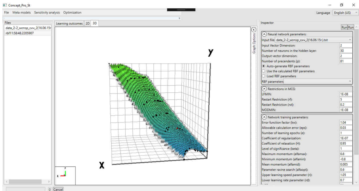
Рис. 4. Визуализация результатов робастной аппроксимации напорных характеристик МОК
