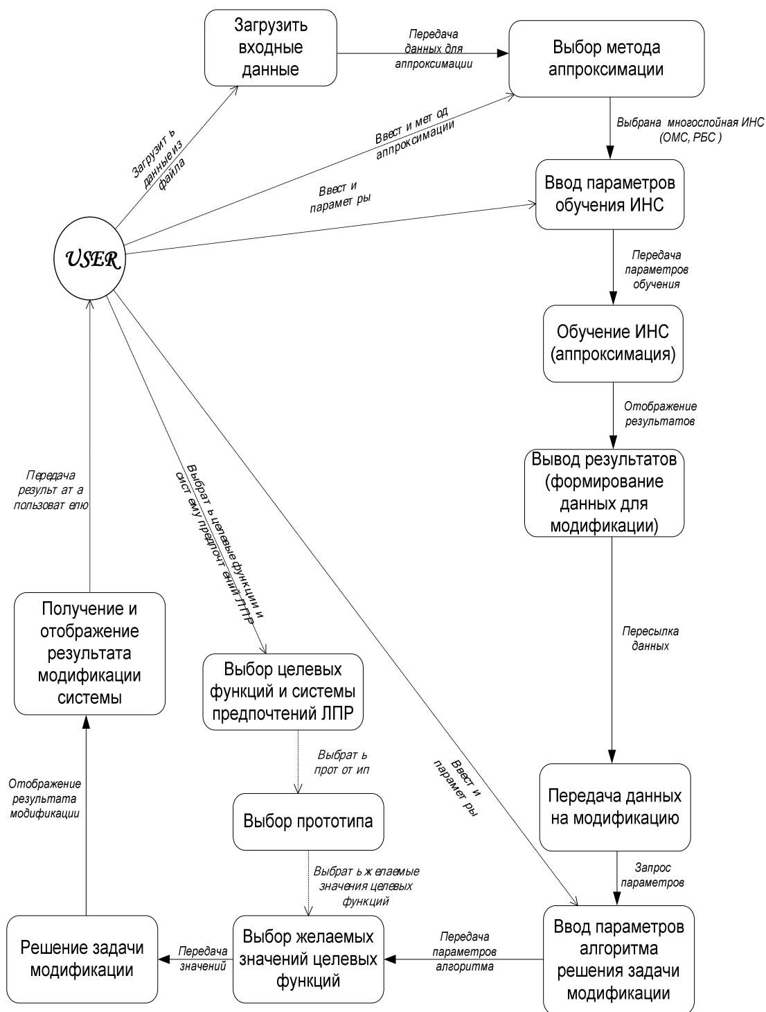
Рис. 1. Контекстная диаграмма процесса принятия решений при формировании облика функционального элемента сложной технической системы
