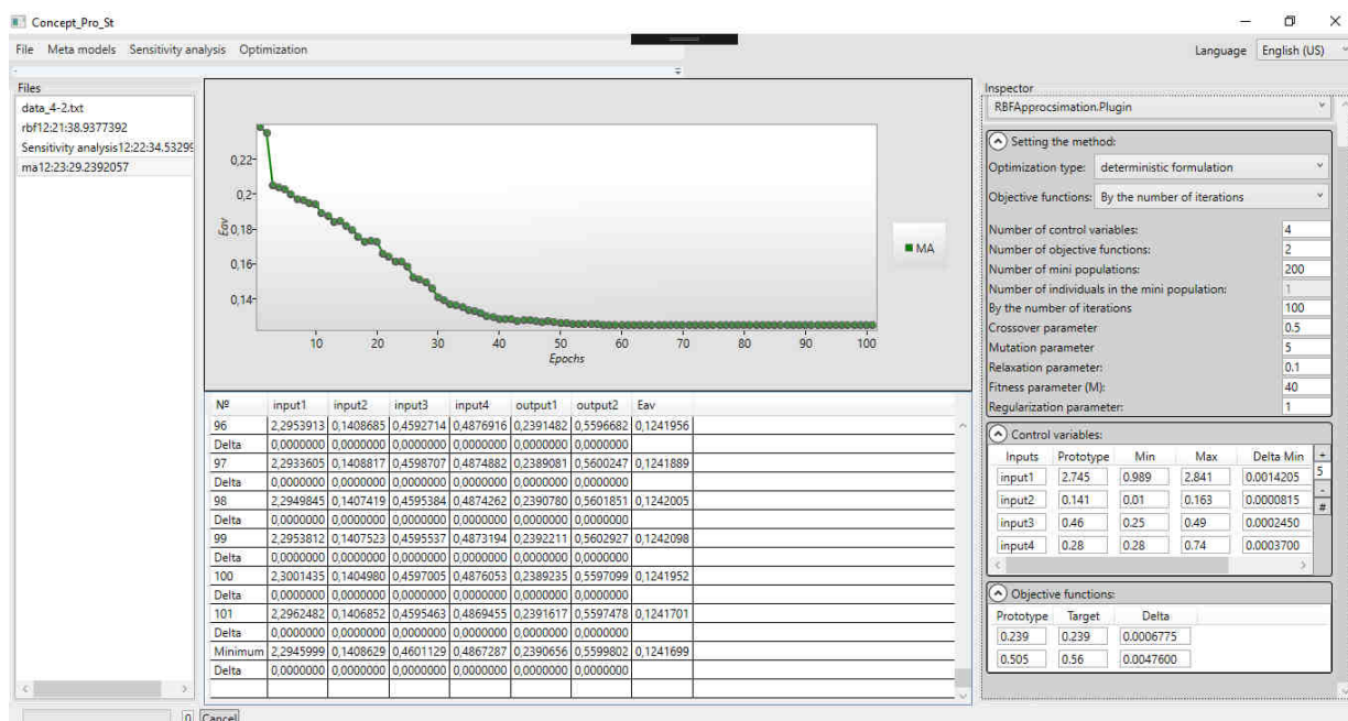
Рис. 6. Пример решения задачи формирования облика промышленного радиального вентилятора в детерминированной формулировке
