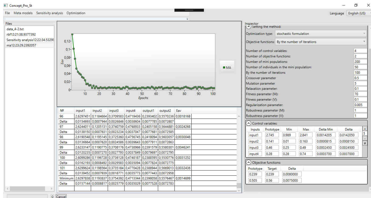
Рис. 7 – Пример решения задачи формирования облика промышленного радиального вентилятора в стохастической формулировке
