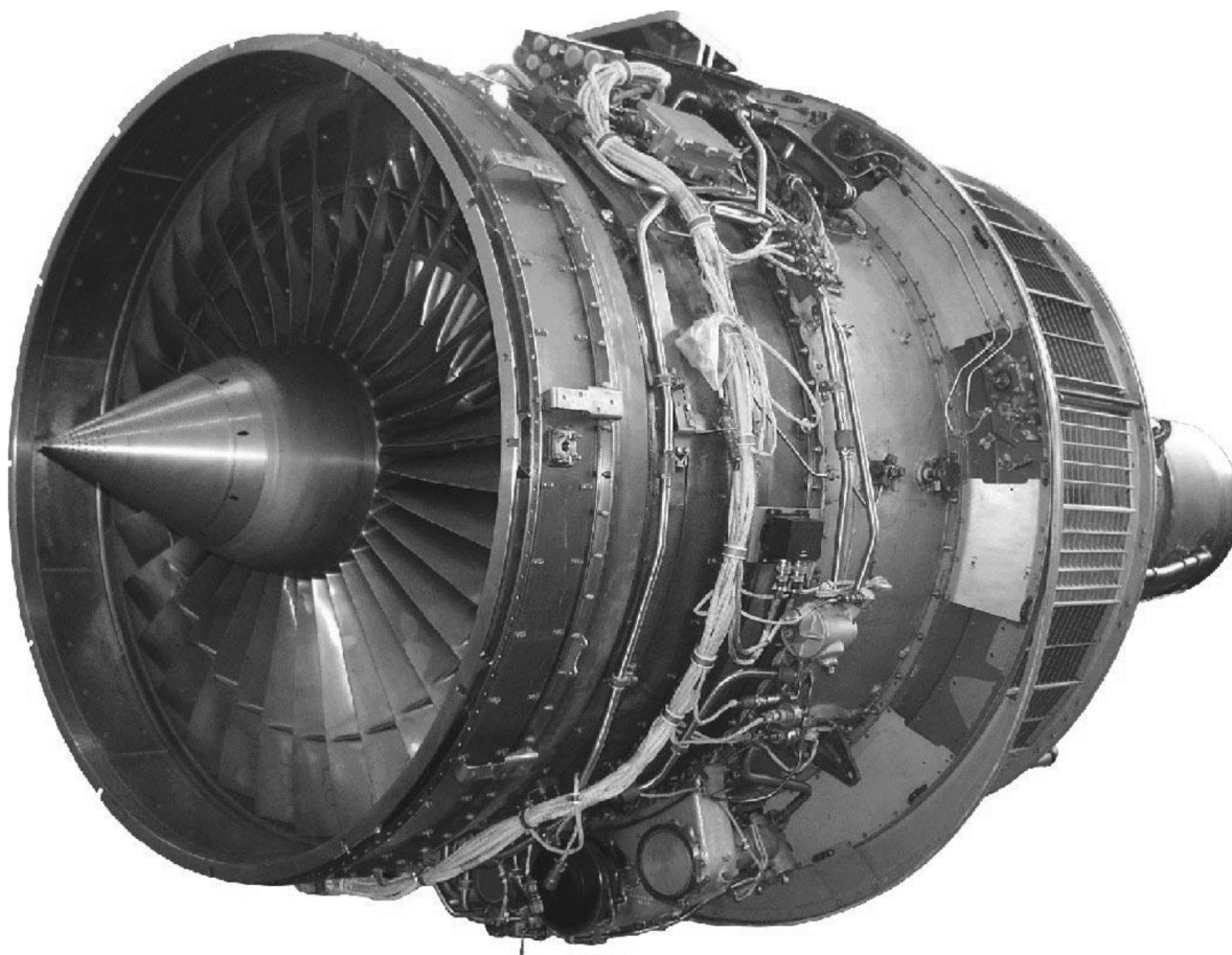
Рисунок 2 – Двигун високого ступеня двоконтурності Д-436-148
