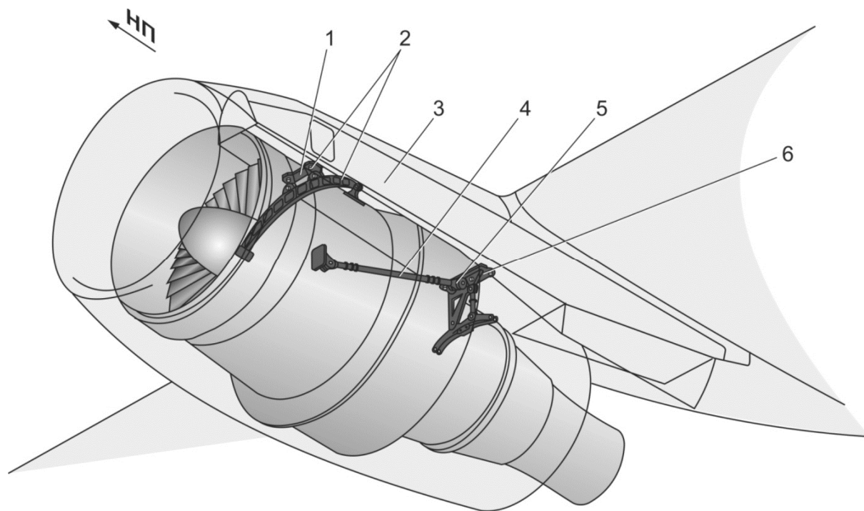
Рисунок 4 – Схема установки двигуна:
