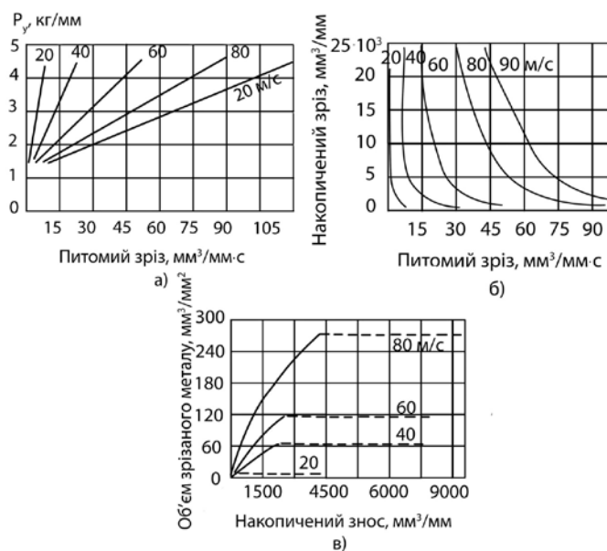
Рис. 1. Результати дослідження процесу швидкісного шліфування композитів при різних швидкостях круга: а – залежність питомої радіальної сили P_r шліфування від питомого зрізу для сплаву 7XG2BMΦ + (4 ÷ 8) % CaF 2 ; б – залежність накопиченого зрізу від питомого зняття шару металу для композиту 11P3AM3Φ2 + (3 ÷ 7) % CaF 2 ; в – залежність об'єму зрізаного металу на одиницю витрат зношеної частини круга від накопиченого об'єму металу для композиту 85X6HΦT + (3 ÷ 8) % CaF 2
