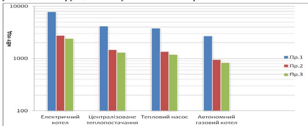
Рис.3. Споживання первинного палива різними джерелами тепла при різних варіантах термічного опору огорожуючих конструкцій: Пр.1 Термічний опір відповідає нормам 80-их років, Пр.2 – відповідає сучасним нормам, Пр.3 – покращений на 20 %.
