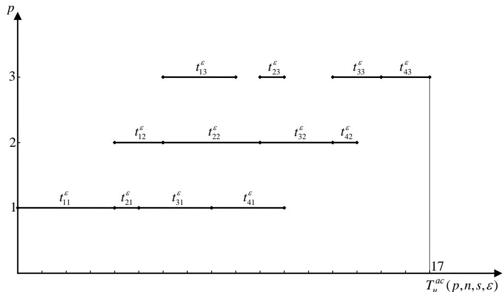
Рис. 1. Асинхронный режим распределенных конкурирующих процессов
