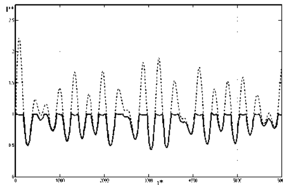
Рис. 2 – Результаты моделирования процесса ограничения мощности при моментном управлении режимом ВЭУ с аэродинамическим мультиплицированием
