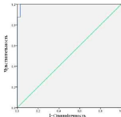
Рис. 1 – ROC-Кривая
