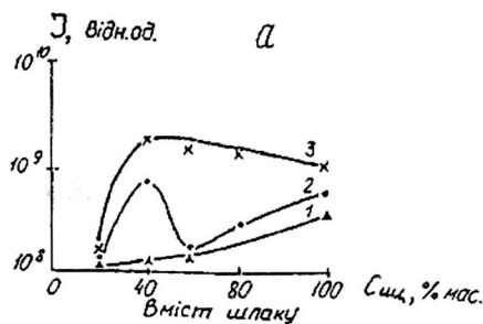
Рис. 3. Зміна інтенсивності (а) і \delta - фактору (б) резонансного сигналу в залежності від вмісту шлаку в системах "вогнестійка глина-шлак феронікелю № 1". 1 – Тобр.=1273К, 2 – 1373К, 3 – 1473К. t_{обр} = 1 год
