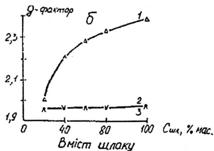
Рис. 3. Зміна інтенсивності (а) і \delta - фактору (б) резонансного сигналу в залежності від вмісту шлаку в системах "вогнестійка глина-шлак феронікелю № 1". 1 – Тобр.=1273К, 2 – 1373К, 3 – 1473К. t_{обр} = 1 год
