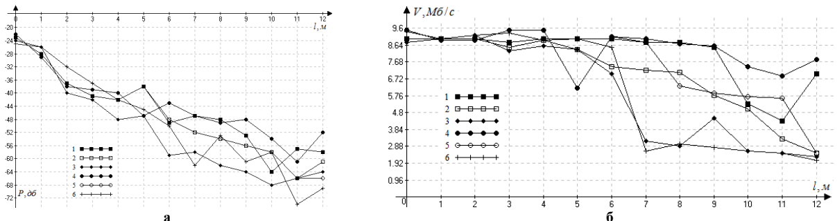
Рис. 3. Залежність швидкості передачі а) та потужності на вході приймача б) від відстані для безпроводного каналу без завад
