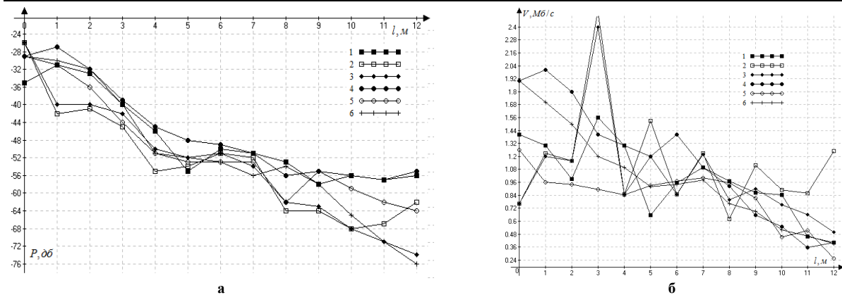
Рис. 7. Залежність швидкості передачі а) та потужності на вході приймача б) від відстані для сусідніх каналів при роботі трьох пристроїв
