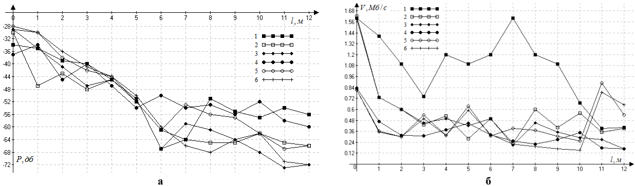
Рис. 5. Залежність швидкості передачі а) та потужності на вході приймача б) від відстані для умов сумісного каналу трьох пристроїв
