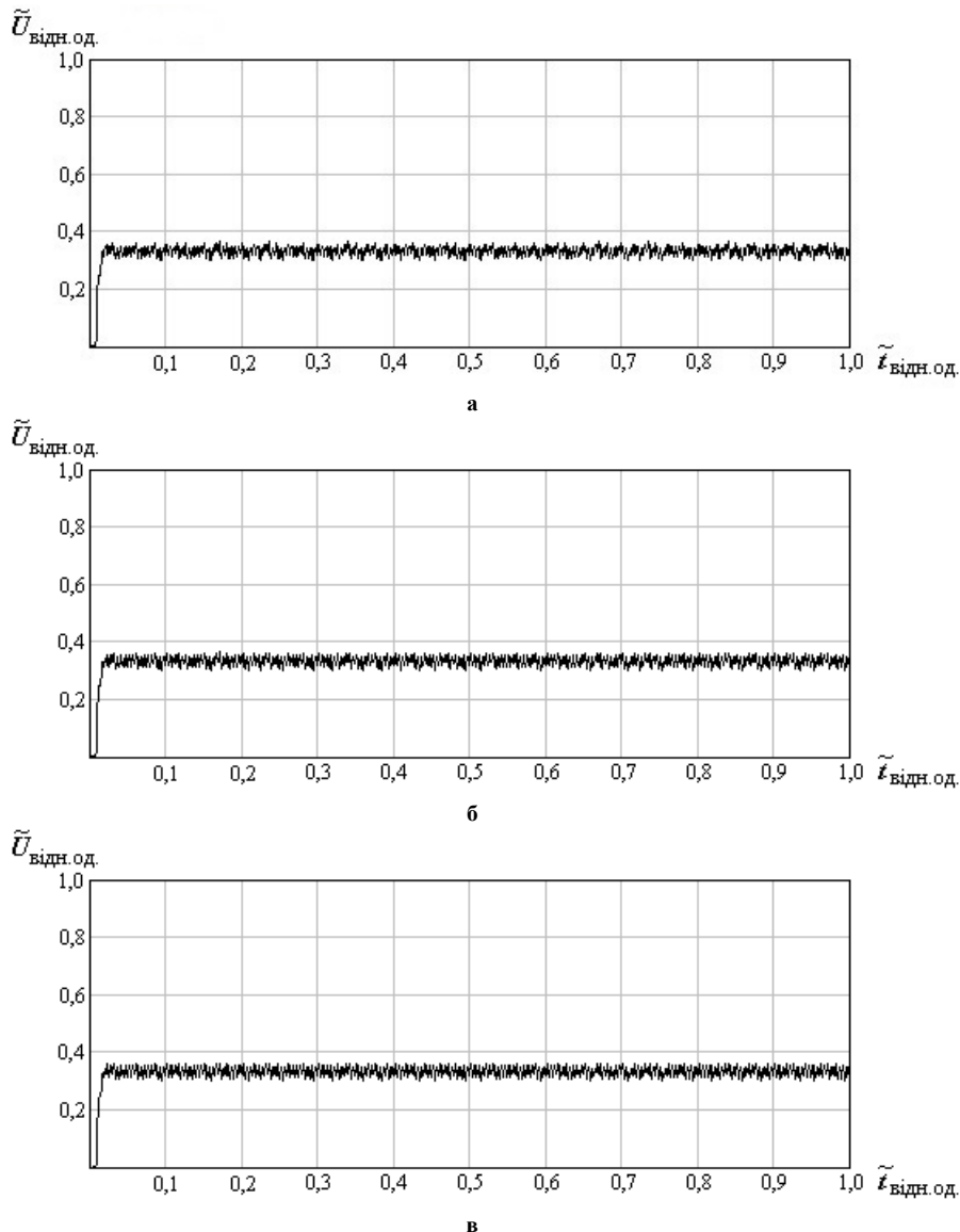
Рис.1. Сигнали АЕ на етапі нормального зношування пари тертя з переважаючим механізмом пластичної деформації при різних значеннях деформацій: а - \varepsilon_{0d} = 11 , б - \varepsilon_{0d} = 15 , в - \varepsilon_{0d} = 19
