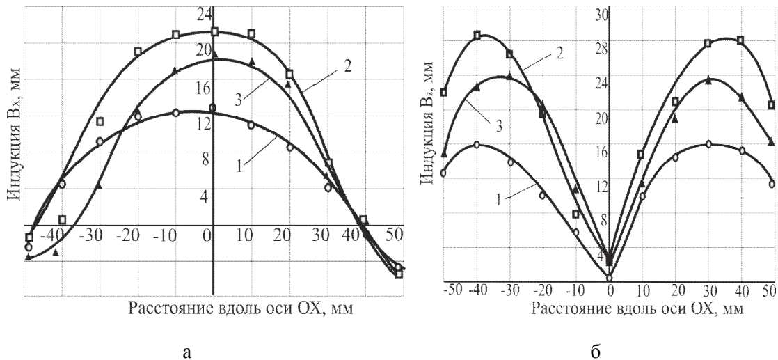
Рис. 2 – Распределение индукций B_x (а), B_z (б) вдоль оси OX ( h = 15 мм; a = 40 мм; H = 35 мм): 1 – с переключкой по рис. 1,в; 2 – с переключкой по рис. 1,б; 3 – без переключки по рис. 1,а
