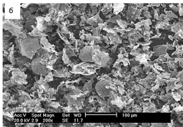
Рис. 2. Мікросвіттлини нанокристалів \text{MgFe}_2\text{O}_4 , які отримані за допомогою скануючого електронного мікроскопу: а – зразок, який отриманий методом співосадження за 873 К; б – зразок, який отриманий золь-гель-методом за 873 К [13].
