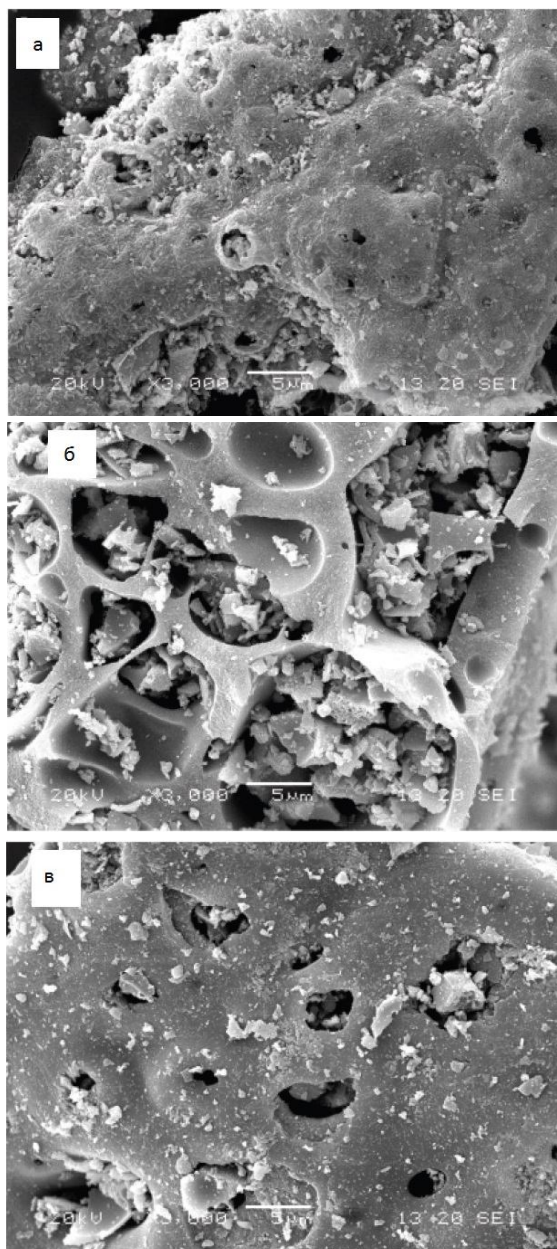
Рис. 3. Мікросвіттлини наночастинок \text{MnFe}_2\text{O}_4 , які отримані за допомогою скануючого електронного мікроскопу. Синтез проведено за температур: а – 673 К; б – 773 К; в – 873 К [14].
