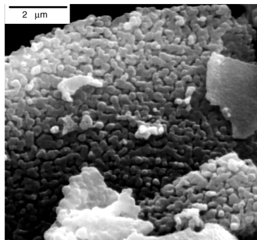
Рис. 9. Мікросвітлина наночастинок \text{MgFe}_2\text{O}_4 , синтезованих за температури 1273 К, яка отримана за допомогою скануючого електронного мікроскопу [28].
