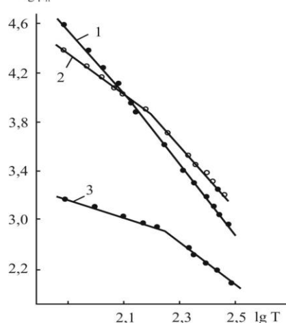
Рис. 14. Температурна залежність холлівської рухливості \mu_n у плівках PbSe на підкладках ВаF 2 (1,2) і ПМ-1 (3) (о - р-тип; • - n-тип провідності).
