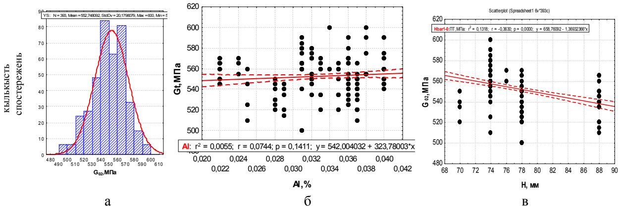
Рис. 1 – Експериментальне частотне розподілення \sigma_{02} (а) та кореляційні залежності \sigma_{02} від технологічних параметрів: б – вмісту Al; в – товщини підкату після червоної кліти (H)
