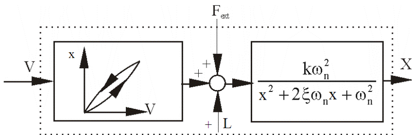
Рисунок 2 – Каскадная модель пьезоелектрического привода
