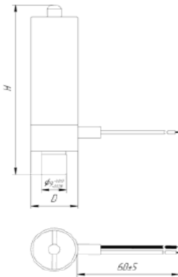
Рисунок 1 – Схема пьезоелектрического актуатора модели АП-К 20/2
