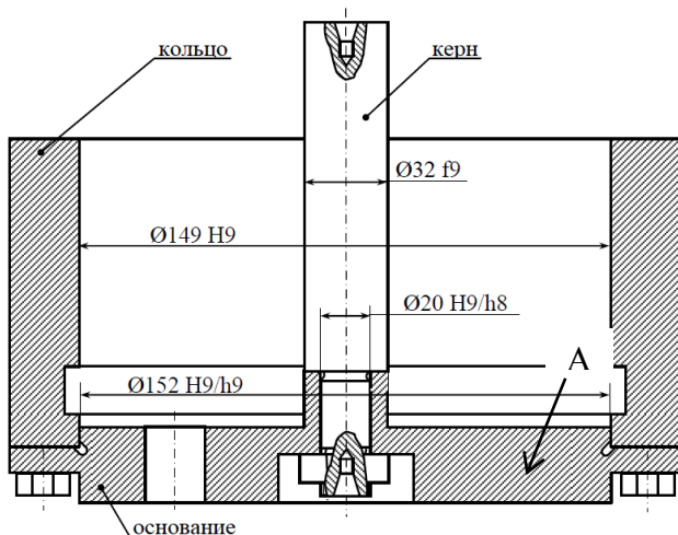
Рисунок 3 – Сборная деталь пресс-формы «основание – kern – кольцо»
