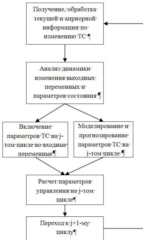
Рисунок 1 – Алгоритм мониторинга процессом шлифования по априорной и динамике изменения текущей информации
