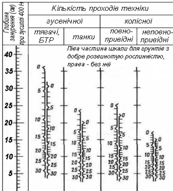
Рис. 4. Номограма визначення проходності місцевості за даними пенетрометра
