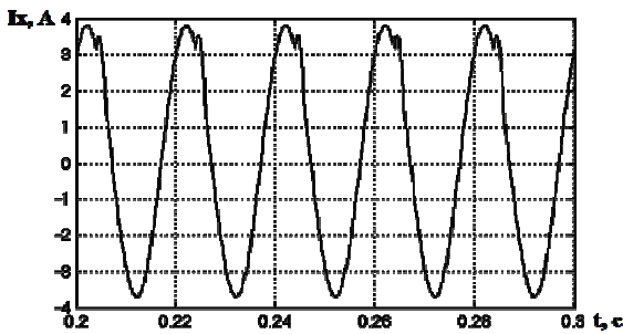
Рис. 4. Крива струму неробочого ходу для значення поверхневої індукованої напруги U = 3 В/км
