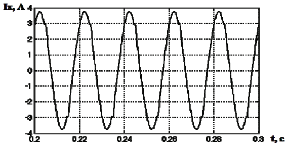
Рис. 2. Крива струму неробочого ходу для значення поверхневої індукованої напруги U = 0 В/км
