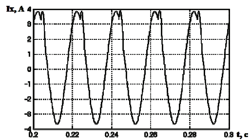
Рис. 5. Крива струму неробочого ходу для значення поверхневої індукованої напруги U = 5 В/км
