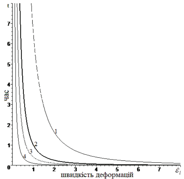
Рис. 2. Гранична крива стаціонарного деформування (2 — розрахунок за (4), n = B = 0,5 ) та криві нестаціонарного деформування (1, 3, 4 — розрахунок за (34)) зі сталим рівнем пошкоджень: 1 — d = 4 ; 3 — d = 1 ; 4 — d = 0,5
