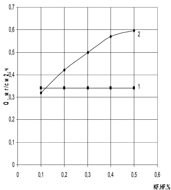
Рис.7. Залежність питомого знімання металу сталі 12X18H10T у розчинах електролітів, режим обробки: A=1,2 мм; f=53 Гц; 1 - \text{HNO}_3 (1,4%)+ \text{HCl} (0,6%); 2 - \text{HNO}_3 (1,4%)+ \text{HCl} (0,6%)+ \text{KF}\cdot\text{HF}
