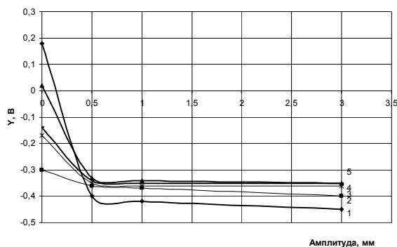
Рис. 1. Залежність потенціалу сталі 12X18H10T від вмісту речовин в розчині: 1 – 0,5% розчин \text{Na}_2\text{SO}_4 ; 2 – 0,5н розчин \text{HCl} ; 3 – 0,5н розчин \text{HNO}_3 ; 4 – 0,5н розчин \text{H}_2\text{SO}_4 ; 5 – 0,5н розчин \text{H}_3\text{PO}_4
