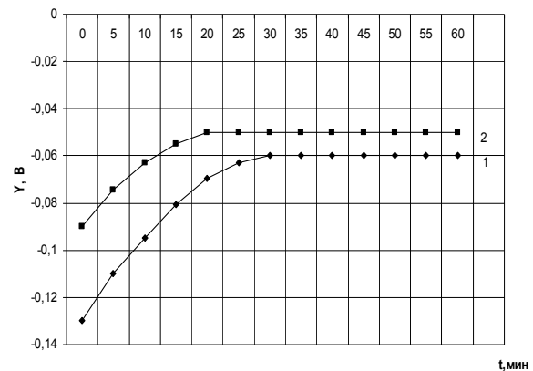
Рис.4. Зміна потенціалів сталі 12X18H10T після припинення дії механічного чинника в часі: 1 – рН = 2; 2 – рН = 2,2
