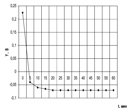
Рис. 3. Зміна потенціалів сталі 12X18H10T у часі в статичних умовах при рН розчину нітратної кислоти 2,4
