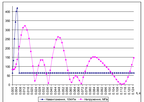
Рис. 7. Зміна еквівалентних напружень \sigma_i
