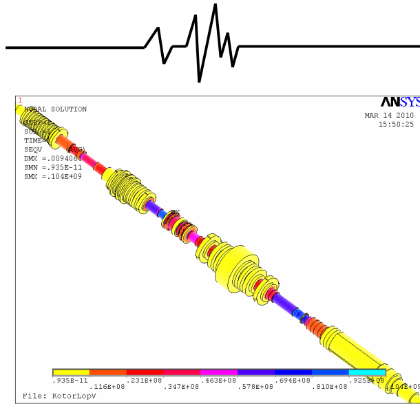
Рис. 3. Схема розподілу інтенсивності напружень по довжині валопроводу у момент часу 0,015с
