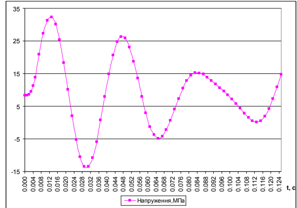
Рис. 5. Зміна дотичних напружень \tau_{yz}
