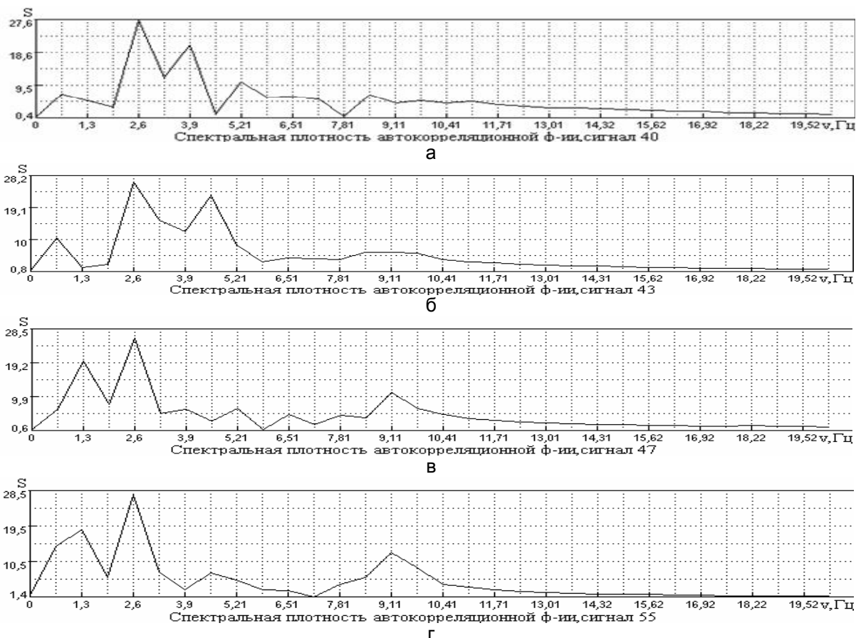
Рис. 1. Спектральные плотности автокорреляционных функций сигналов потребляемой мгновенной мощности привода мельниц в зависимости от степени заполнению: а – 40%; б – 43%; в – 47%; г – 55%
