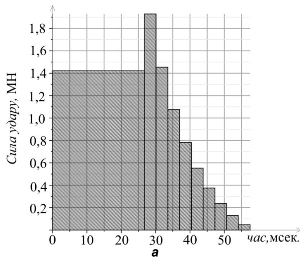
Рис. 1. Діаграма ударного імпульсу для двох компонентів БК в зоні прихоплення
