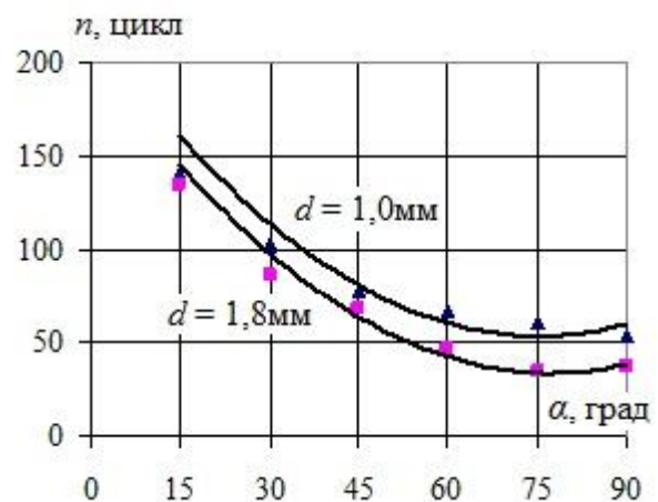
Рис. 6. Залежності стійкості дробу n від кута атаки \alpha для фракцій діаметра d
