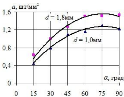
Рис. 7. Залежності ступеня шаржування a від кута атаки \alpha для фракцій діаметра d
