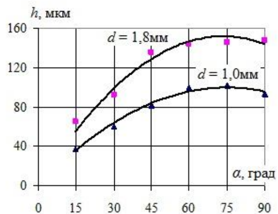
Рис. 8. Залежності глибини рельєфу h від кута атаки \alpha для фракцій діаметра d
