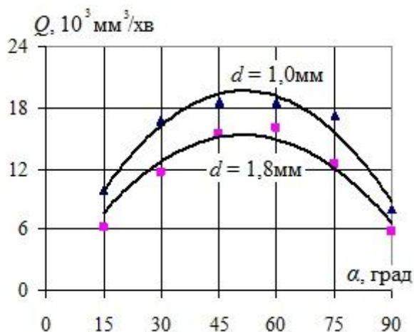
Рис. 5. Залежність продуктивності Q від кута атаки \alpha для фракцій діаметра d
