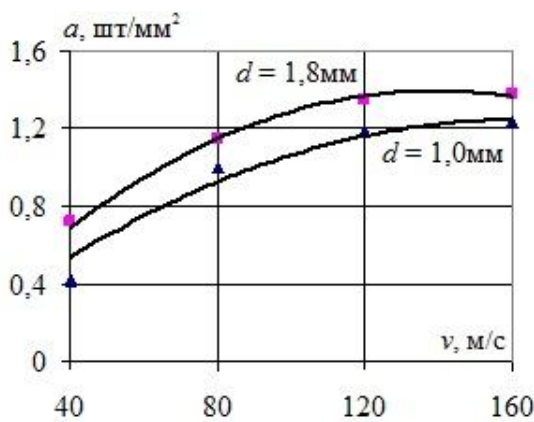
Рис. 3. Залежності ступеня шаржування a від швидкості атаки v для фракцій діаметра d
