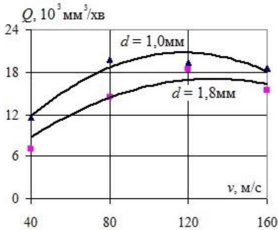
Рис. 1. Залежність продуктивності Q від швидкості атаки v для фракцій діаметра d
