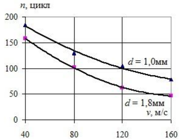
Рис. 2. Залежності стійкості дробу n від швидкості атаки v для фракцій діаметра d
