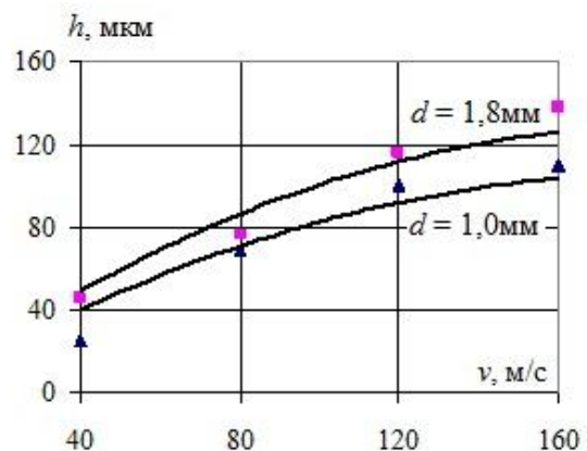
Рис. 4. Залежності глибини рельєфу h від швидкості атаки v для фракцій діаметра d
