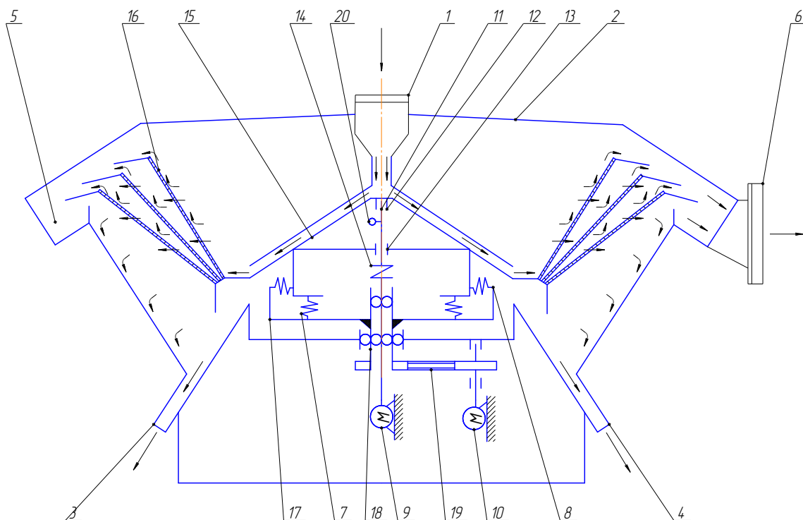
Рис. 2. Вібраційна центрифуга з дебалансним приводом: 1 – завантажувальна горловина; 2 – корпус; 3,4 – вивантажувальні патрубки відфільтрованого матеріалу; 5 – відділення для осаду; 6 – вивантажувальна горловина осаду; 7, 8 – пружні елементи; 9, 10 – електродвигун; 11 – приводний вал незрівноважених мас; 12, 13 – підшипникові вузли; 14 – гнучка муфта; 15 – приводний конус; 16 – фільтраційні елементи; 17 – приводна платформа; 18 – приводний вал платформи; 19 – клинопасова передача; 20 – дебаланс
