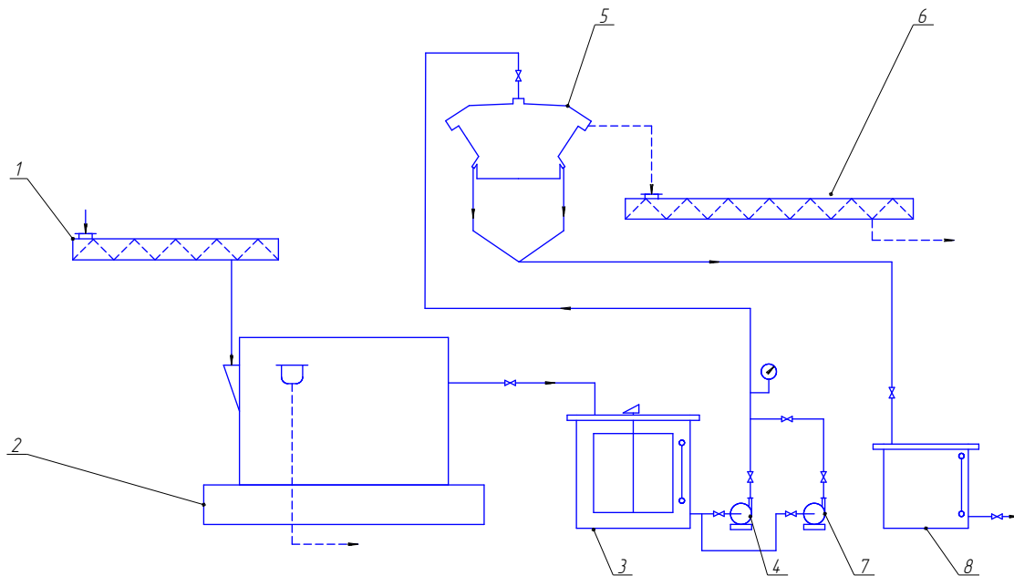
Рис. 1. Технологічна схема первинного очищення соняшникової пресової олії: 1 – шнек; 2 – механічна пастка; 3 – збірник для олії; 4,7 – насос; 5 – центрифуга; 6 – бак для олії; 7 – шнек
