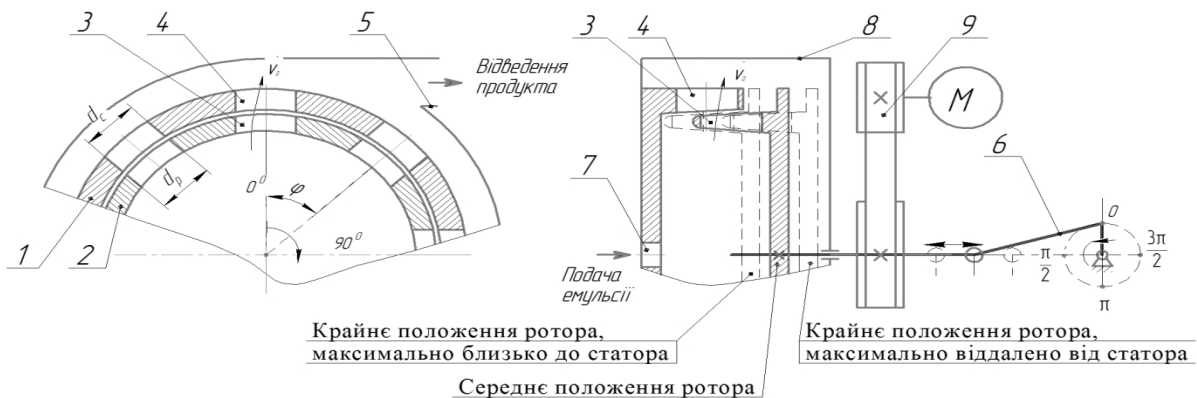
Рис. 4. Схема роторно-пульсаційного гомогенізатора з ротором, що вібрує
