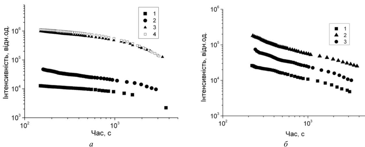
Рис. 1. Кінетика спаду фосфоресценції кристалів \text{CaF}_2 , опроміненних інтегральними потоками електронів: а – 10^{11} \text{ см}^{-2} (крива 1), 5 \cdot 10^{11} \text{ см}^{-2} (крива 2), 2 \cdot 10^{12} \text{ см}^{-2} (крива 3), 5 \cdot 10^{12} \text{ см}^{-2} (крива 4); б – 10^{14} \text{ см}^{-2} (крива 1), 8 \cdot 10^{16} \text{ см}^{-2} (крива 2), 3 \cdot 10^{17} \text{ см}^{-2} (крива 3).
