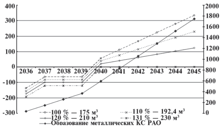
Рис. 2. Пример определения оптимальной переработки (дезактивации) металлических отходов в зависимости от различных производительностей установок дезактивации в период с 2036 по 2045 гг.
