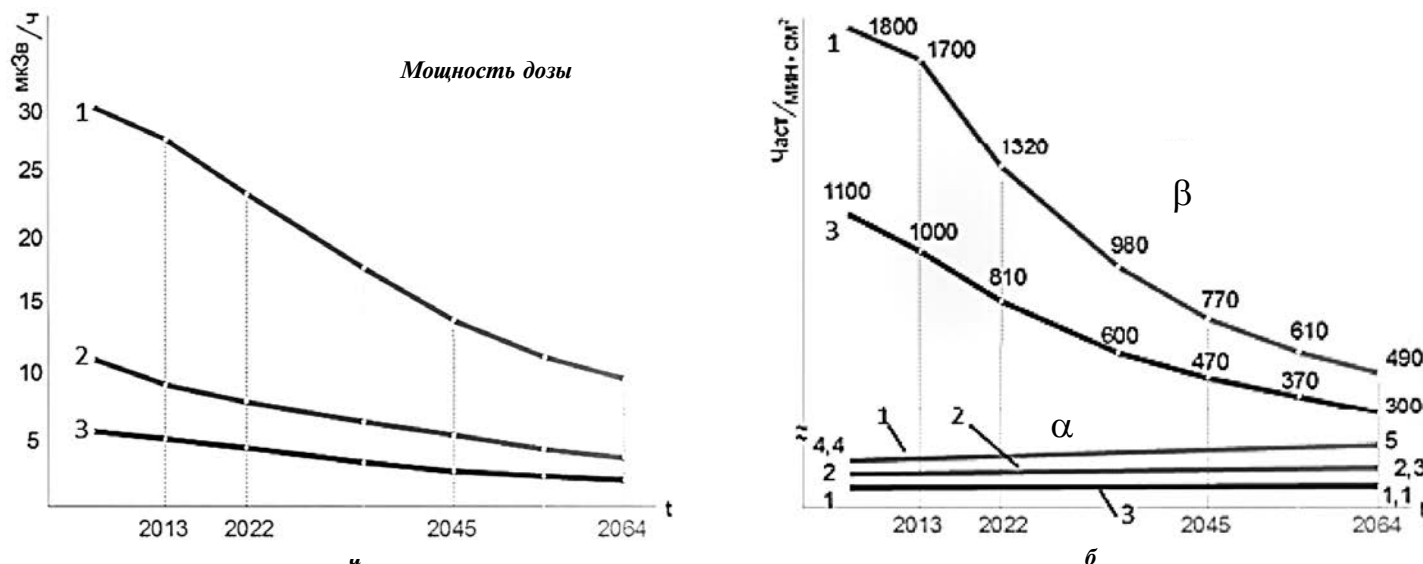
Рис. 4. Критерии группы 2 для помещений ограниченного обслуживания (1), полуобслуживаемых помещений (2), обслуживаемых помещений (3): а — мощность дозы на расстоянии 1 м; б — плотность поверхностного загрязнения
