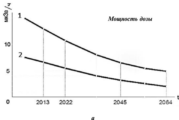
Рис. 3. Критерии группы 1 для территорий усиленного контроля (1) и свободного режима (2): а — мощность дозы на расстоянии 1 м; б — плотность поверхностного загрязнения
