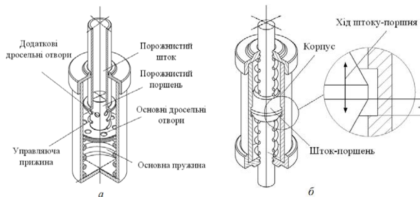
Рис.1 – Пасивні демпфери: при реалізації перекриття дросельних отворів (а); при реалізації змінного дросельного отвору у вигляді проміжку між штоком-поршнем та циліндром амортизатора (б)
