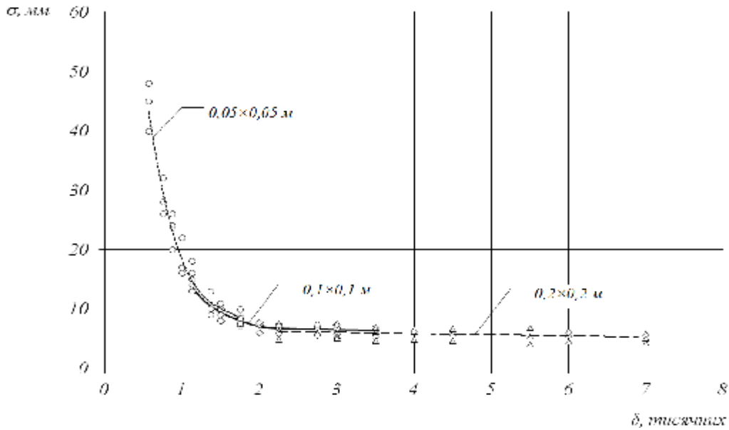
Рис. 4 – Залежність СКВ координат наведення прицілу Leupold Mark 4 від уявних кутових розмірів цілі
