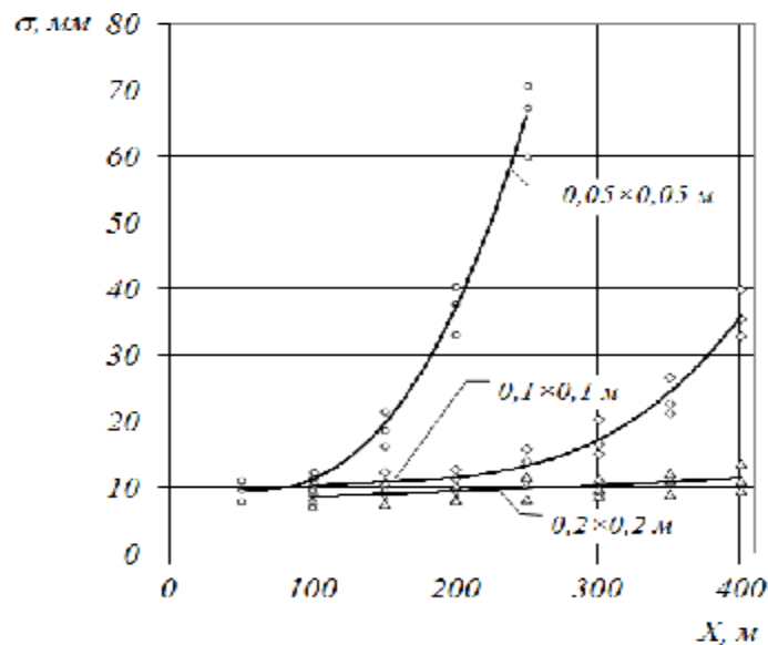
Рис. 3 – Залежність СКВ координат наведення прицілу ПСО-1 від дальності до цілі
