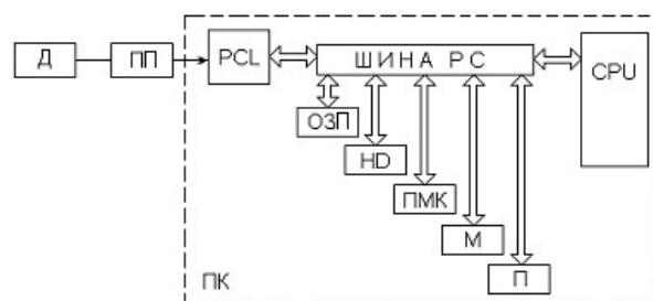
Рисунок 1 – Загальна структура побудови акусто-емісійної системи для діагностики пар тертя: Д – датчик; ПП – попередній підсилювач; PCL – порт введення виведення інформації; ОЗП – оперативний запам'ятовуючий пристрій; HD – жорсткий диск; ПМК – програмний математичний комплекс; М – монітор; П – принтер; CPU – процесор; ПК – персональний комп'ютер.
