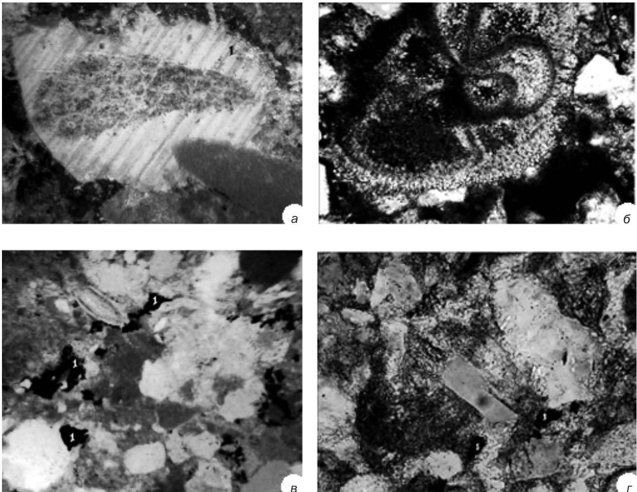
Рис. 2. Зони регенерації карбонату та виділення вуглецевої речовини у цементі пісковиків
